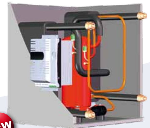
EM III i , Sole/Wasser Querschnitt EM III i , Brine/Water cross sectional view
