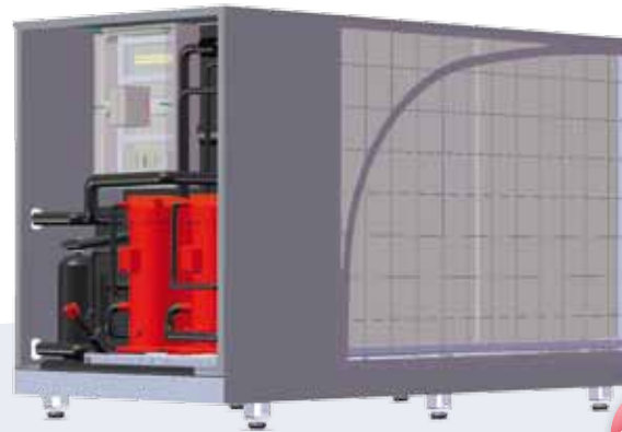
aero 050 - 080 Querschnitt cross sectional view
